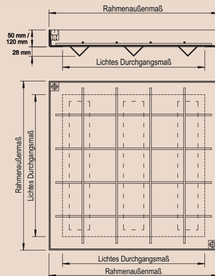
Stahl feuerverzinkt
